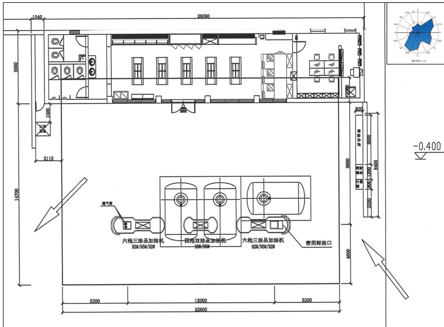
附图3 项目总平面布置图 (1:200)
