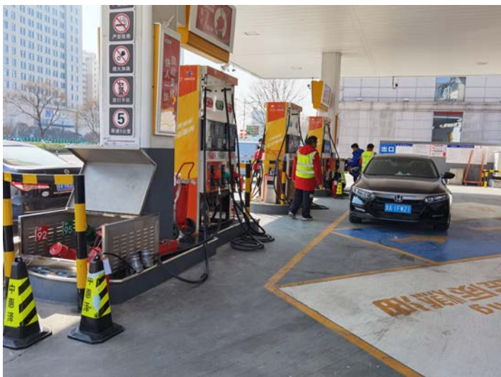
二次油气回收
